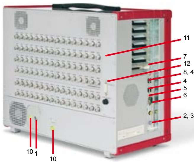
Typische DEWE-4011 Rückseite
