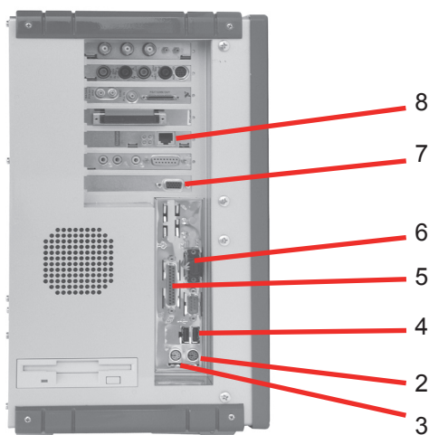
Typische DEWE-4018 Seitenansicht
