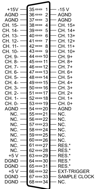
68 pol. Stecker
