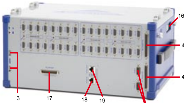
Typische DEWE-511 Vorderseite
