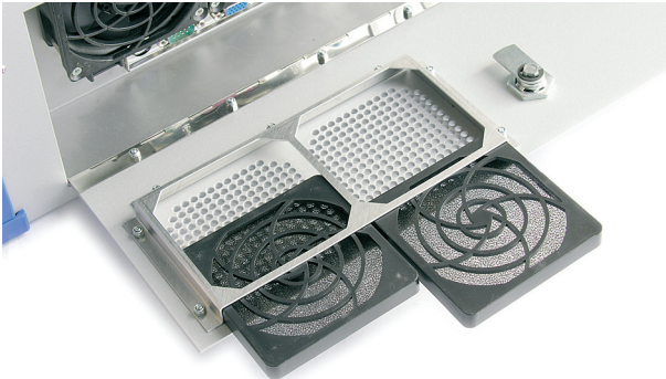
Filterschublade mit Filter
