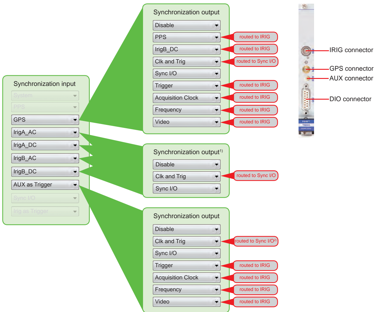
TRION-TIMING module
