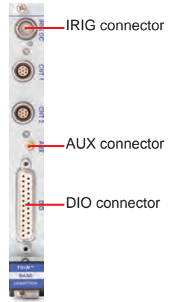
TRION-BASE module
