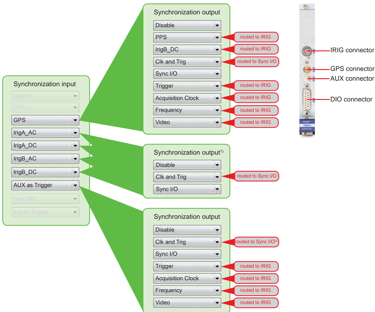
TRION-TIMING module
