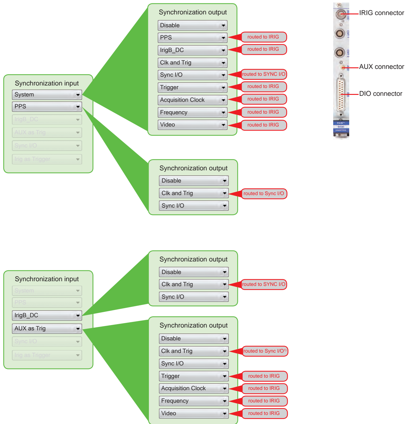
TRION-BASE module
