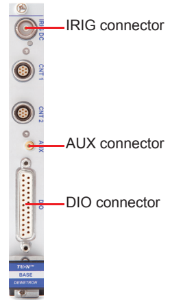
TRION-BASE module
