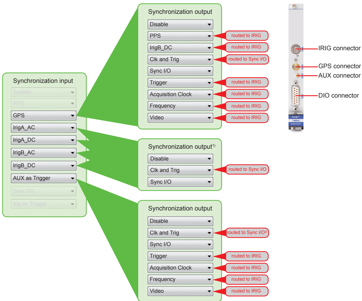
TRION-TIMING module
